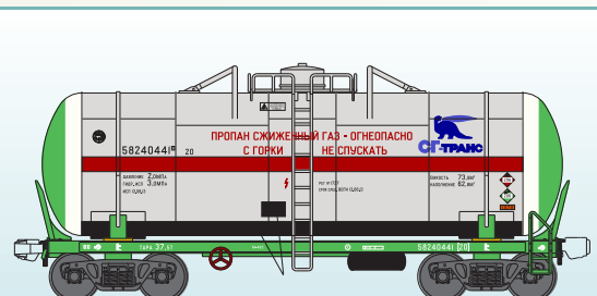
0008 Две цистерны "СГ-Транс" для перевозки сжиженного газа РЖД 0008 Two tank cars for "SG-Trans" for liquefied gas RZD (ep. VI)
